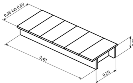
Rys. 4. Geometria półki zapory przeciwybuchowej pyłowej Fig. 4. Geometry of dust explosion - proof firewall shelf
