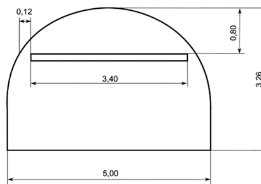
Rys. 5. Położenie półki zapory przeciwybuchowej pyłowej w przekroju wyrobiska górnicy Fig. 5. Dust explosion-proof firewall shelf placement in cross section of mine drift
