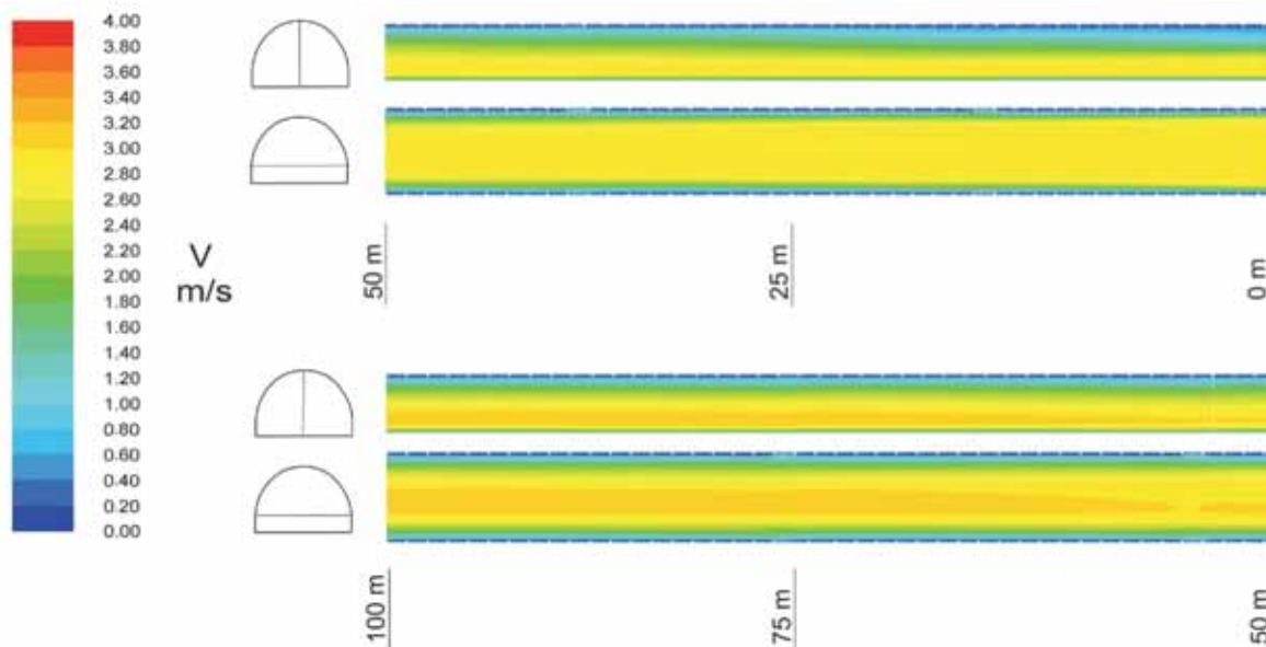
Rys. 9. Kształtowanie się profilu prędkości za zaporą pyłową
