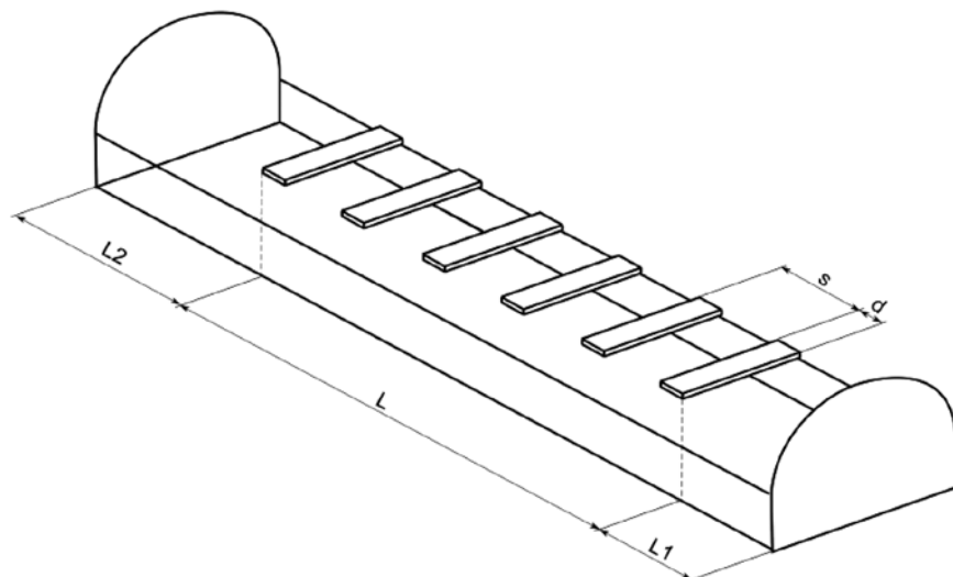
Rys. 6. Geometria zapory przeciwybuchowej pyłowej w wyrobisku górnicy Fig. 6. Geometry of dust explosion-proof firewall in the mine drift
