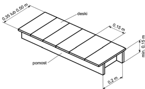
Rys. 2. Wytyczne konstrukcji półki zapory przeciwwybuchowej pyłowej [7]
