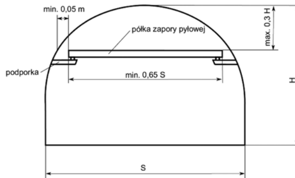
Rys. 3. Wytyczne położenia półki zapory przeciwwybuchowej pyłowej w przekroju wyrobiska górniczego [7]
