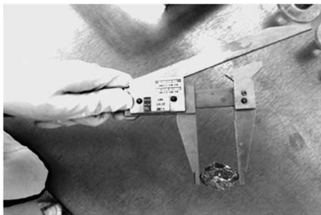
Rys. 2. Sprawdzenie kształtu ziarna
