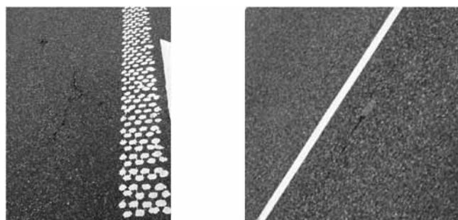
Rys. 3. Spękania zmęczeniowe poza obszarem uskoku (fot. M. Grygierek)
