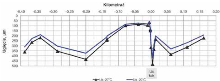
Rys. 15. Ugięcia nawierzchni – przypadek C Fig. 15. Pavement deflection – case C Źródło: opracowanie własne
