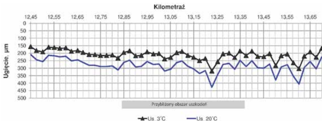
Rys. 9. Ugięcia sprężyste nawierzchni – przypadek B
