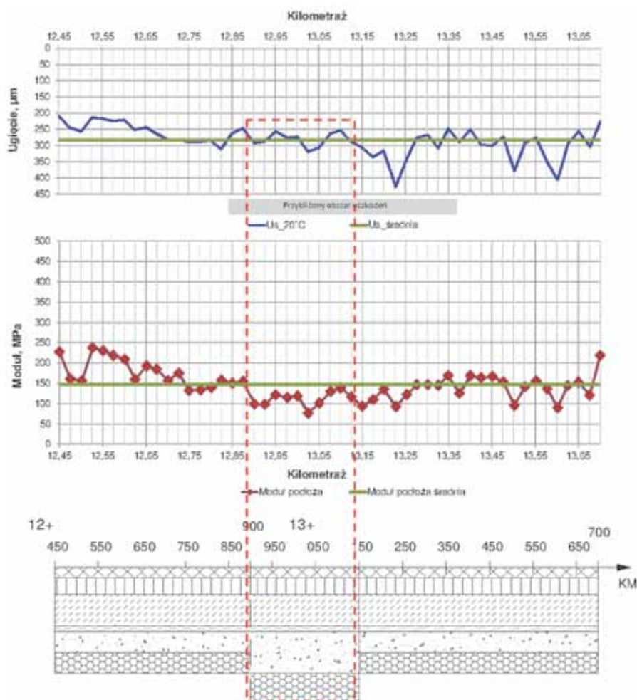
Rys. 17. Zestawienie wyników dla przypadku B.
