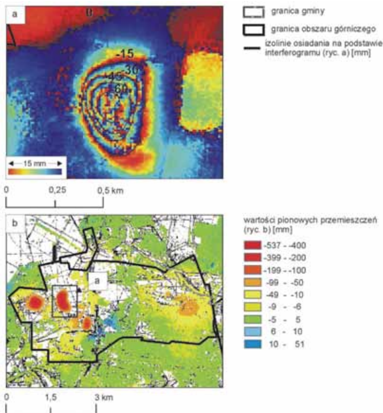
Rys. 4. Opracowanie zbioru punktów zawierającego informacje o pionowych przemieszczeniach terenu na obszarze Bytomia. a. Manualna digitalizacja prążków interferometrycznych na interferogramie z okresu 06.12.2011÷17.12.2011. b. Kompleksowy zbiór punktów przedstawiający zarówno dane PS o niewielkich przemieszczeniach (rys. 2a), jak i punkty o dużych przemieszczeniach zidentyfikowanych na podstawie interferogramów.
