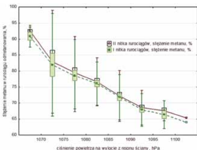
Rys. 17. Zmiany stężenia metanu w rurociągach odmetanowania tzw. I i II nitka rurociągu
