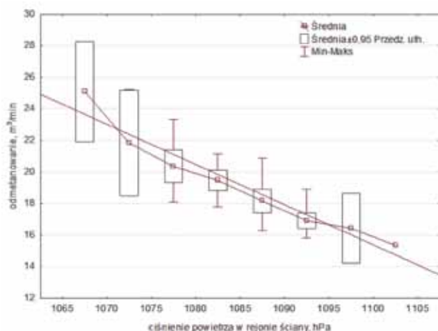
Rys. 16. Zmiany ilości ujętego metanu poprzez odmetanowanie ze ściany 2 pokład 506 w zależności od ciśnienie powietrza w rejonie ściany
