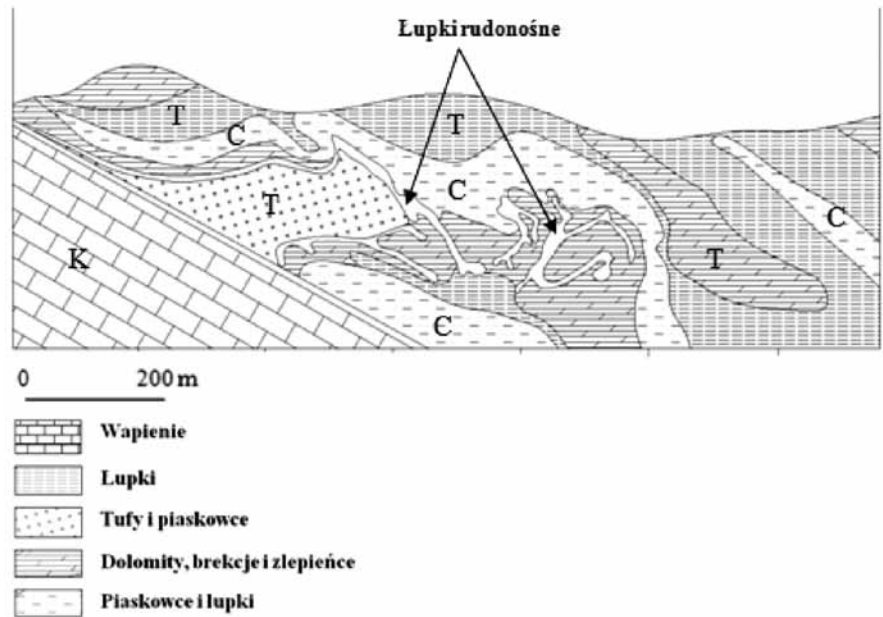
Rys. 2. Przekrój geologiczny przez złożę w rejonie Idriji (uproszczony schemat w oparciu o materiały ze zbiorów Muzeum Geologii Złóż im. Czesław Poborskiego na Wydziale Górnictwa i Geologii Politechniki Śląskiej)
