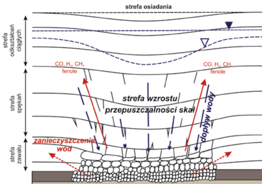
Rys. 2. Osiadanie i spękania nadkładu, deformacje powierzchni terenu, emisja gazów ( \text{CO} , \text{CO}_2 , \text{H}_2 , związków organicznych), możliwe zanieczyszczenie wód podziemnych i atmosfery w związku z eksploatacją węgla metodą podziemnego zgazowania [wg 17, zmodyfikowany]
