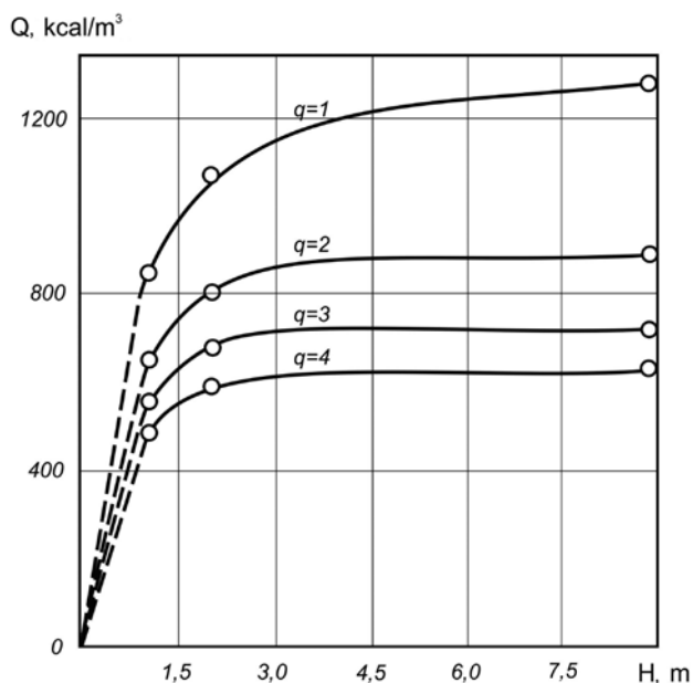
Rys. 1. Zależność wartości opalowej gazu Q (kcal/m 3 ) od miąższości złoże H (m) i dopływu wody q (m 3 /t) [wg. 12]
