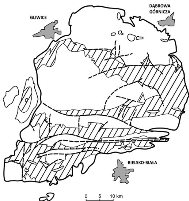
Rys. 7. Obszar występowania pokładu 510 w GZW na głębokości 1000 ÷ 1500 m (zaszraflowany)
