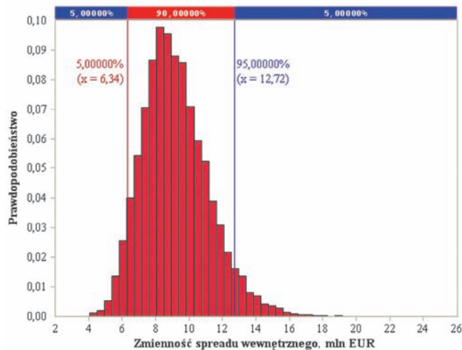
Rys. 3. Histogram symulacji zmienności spreadu wewnętrznego kopalni w oparciu o kontrakty futures month – ceny symulowane niezależnie.
