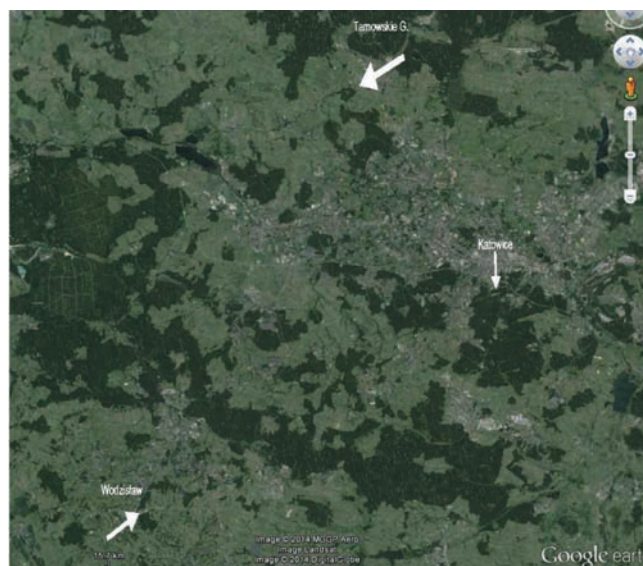
Rys. 3. Wektory przemieszczeń poziomych stacji ASG-EUPOS w GZW (w lokalnym układzie współrzędnych). Objaśnienia w tekście (opracowano na podkładzie Google Earth).
