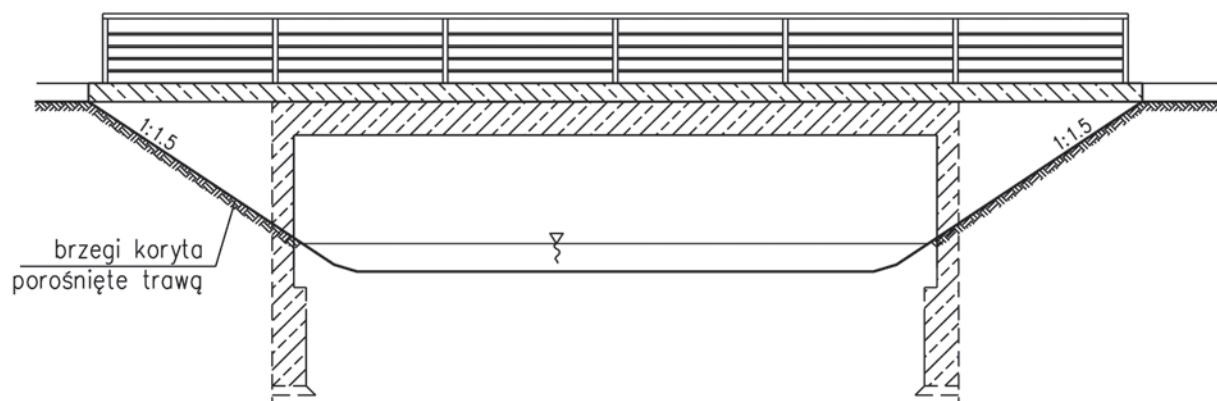
Rys. 4. Most ramowy posadowiony bezpośrednio
