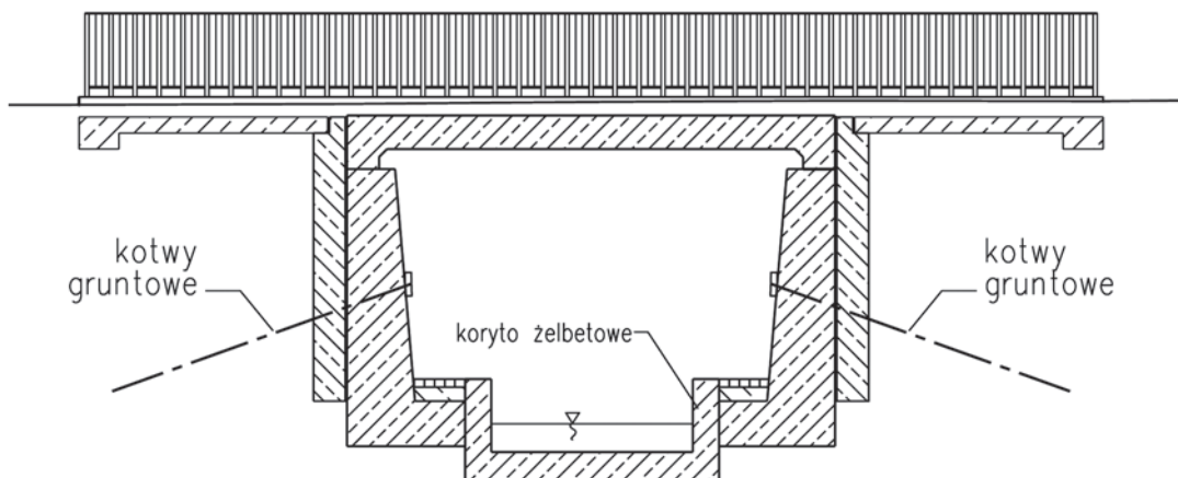
Rys. 9. Most z kintą żelbetową w wyciętej płycie dennej
