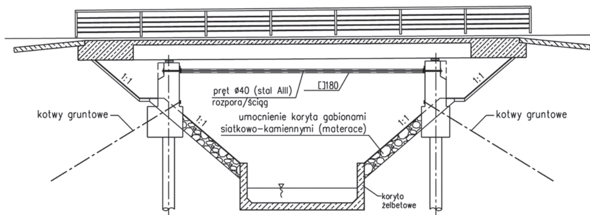
Rys. 3. Most na palach. Znaczne obniżenie dna koryta
