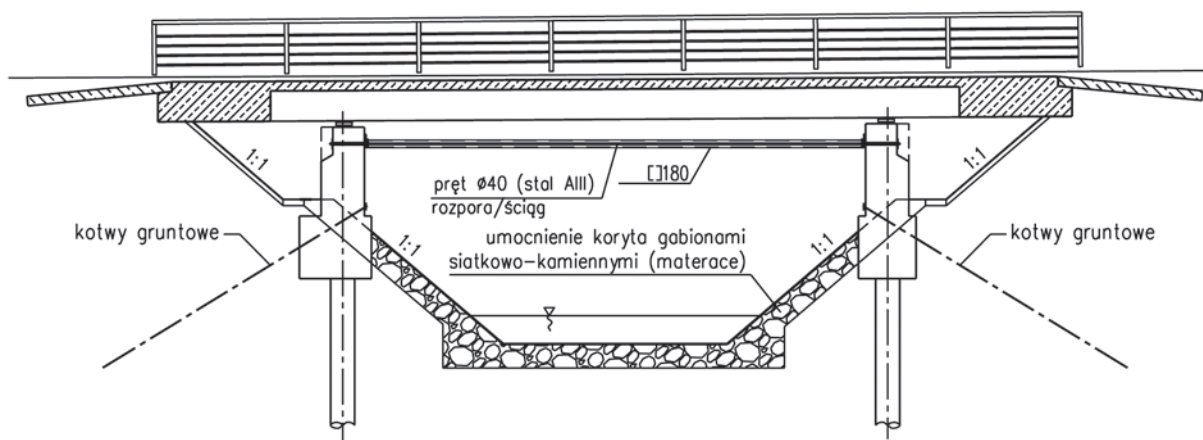
Rys. 2. Most na palach. Umiarkowane obniżenie dna koryta
