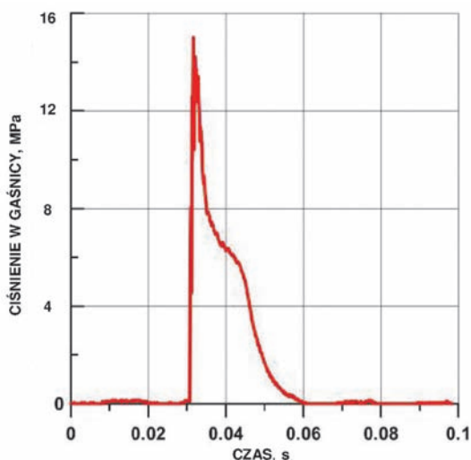
Rys. 5. Przebieg ciśnienia w gaśnicy podczas próby tłumienia wybuchu [5], [2]
