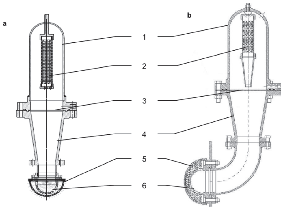
Rys. 1. Schemat gaśnicy testowej o objętości 5 dm 3 (a) oraz 10 dm 3 (b) [5]
