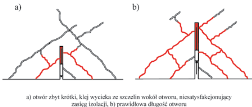
Rys. 3. Dobór odpowiedniej długości otworów iniekcyjnych
