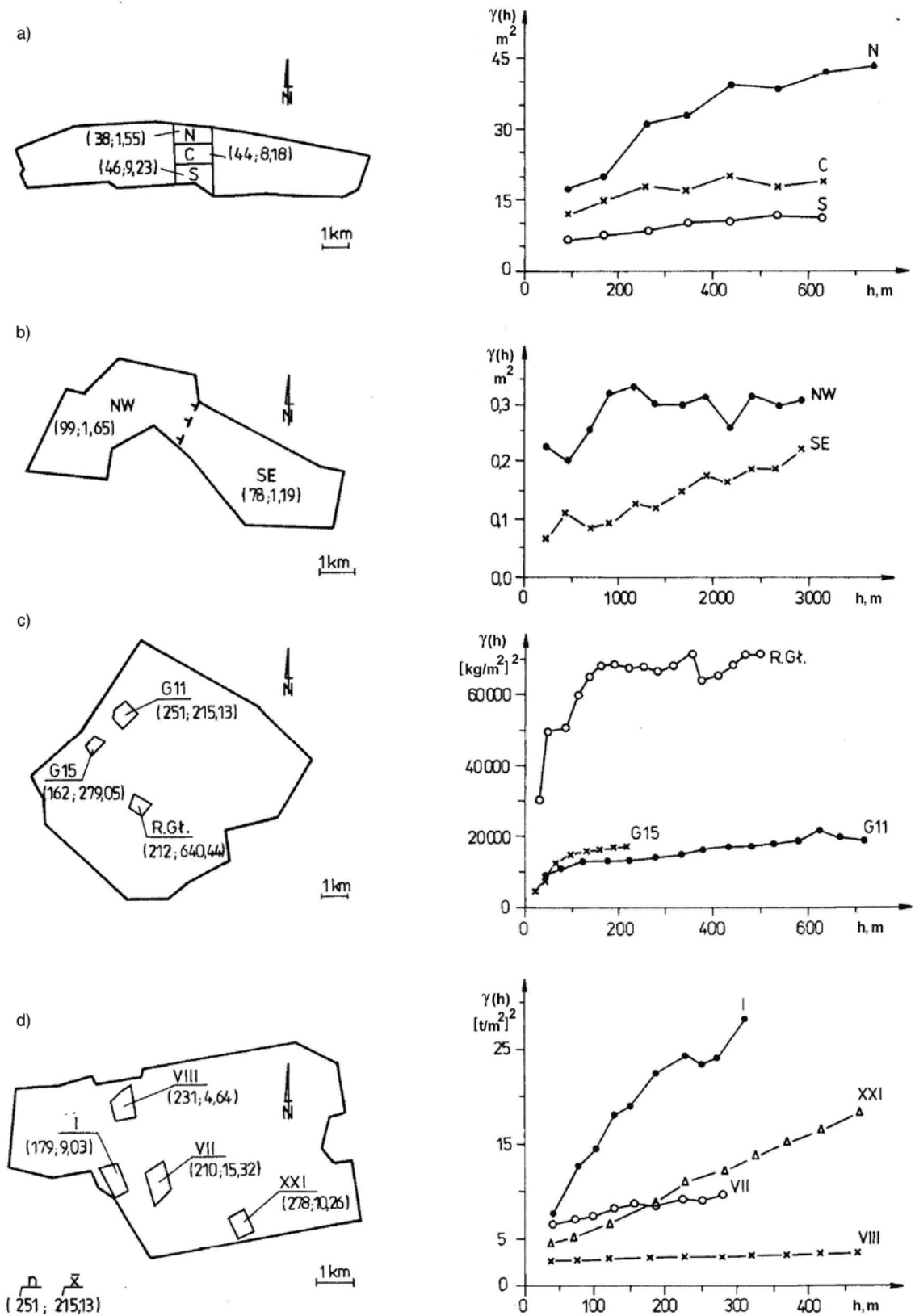
Rys. 5. Przykłady obszarowego zróżnicowania semiwariogramów parametrów złożowych
