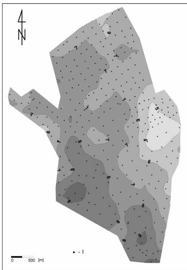
Rys. 3. Mapa izolunii miąższości warstwy kruszywa naturalnego w dolinie Odry sporządzona metodą krzygu zwykłego (obszar badań obejmuje złoża: Lubomia III, Nieboczowy III oraz fragment złoża Racibórz II – zbiornik) [9] 1 – otwory wiertnicze
