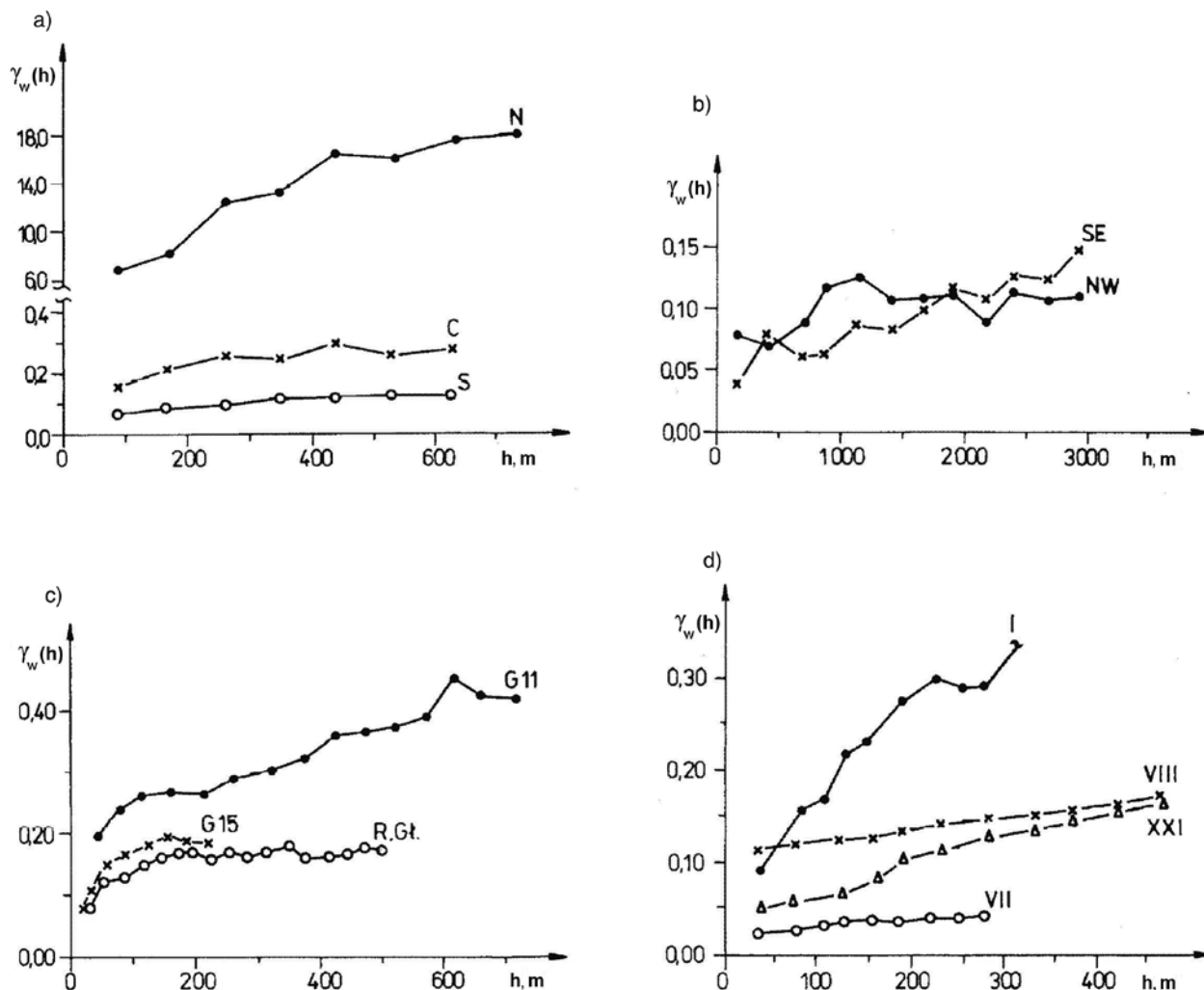
Rys. 8. Badanie efektu proporcjonalności przy pomocy semiwariogramów względnych a) miąższość użyteczna węgla w poziomie V KWB Belchatów, b) miąższość pokładu węgla 407/1 w KWK Staszic, c) zasobność Cu w złożu rud miedziowo-srebrowych kopalni Rudna, d) zasobność złoża siarki rodzimej Jeziórko; N, NW, G15, VII – wydzielone części złoża przedstawione na rys. 5.
