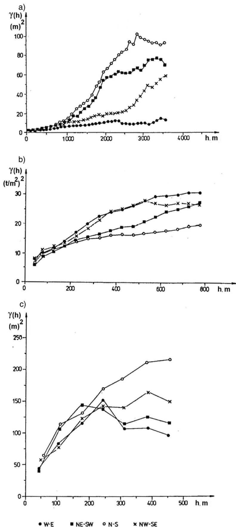
Rys. 1. Semiwariogramy ukazujące występowanie anizotropii zmienności parametrów złożowych na większych obszarach [9]
