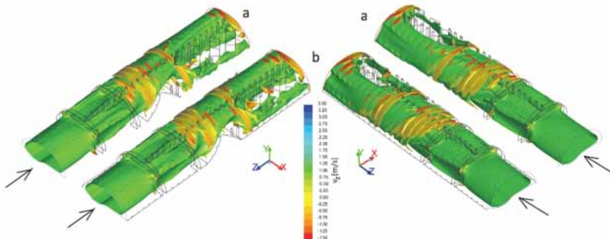
Rys. 15. Porównanie izopowierzchni prędkości 1.0 m/s, a - stan pierwotny, b - po ułożeniu przeszkody na spągu Fig. 15. Comparison of isosurface for 1.0 m/s velocity, a - state before, b - state after floor bulge
