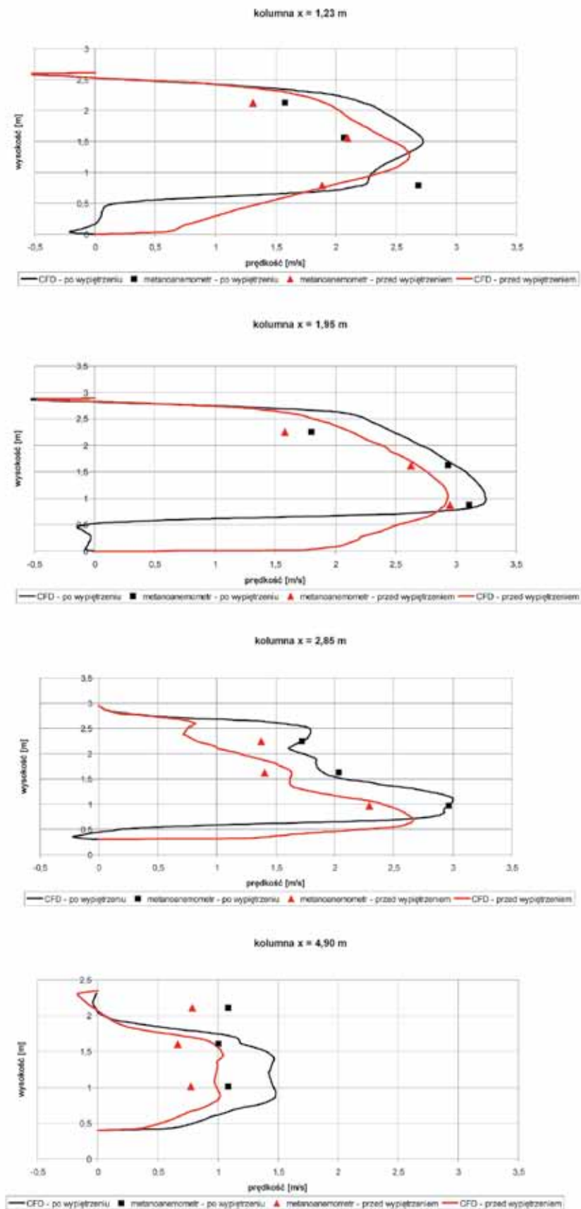
Rys. 6. Porównanie wyników symulacji z punktowymi pomiarami prędkości dla stanów przed i po ułożeniu worków Fig. 6. Comparison of simulation results with velocity measurements in points for the states before and after floor bulge
