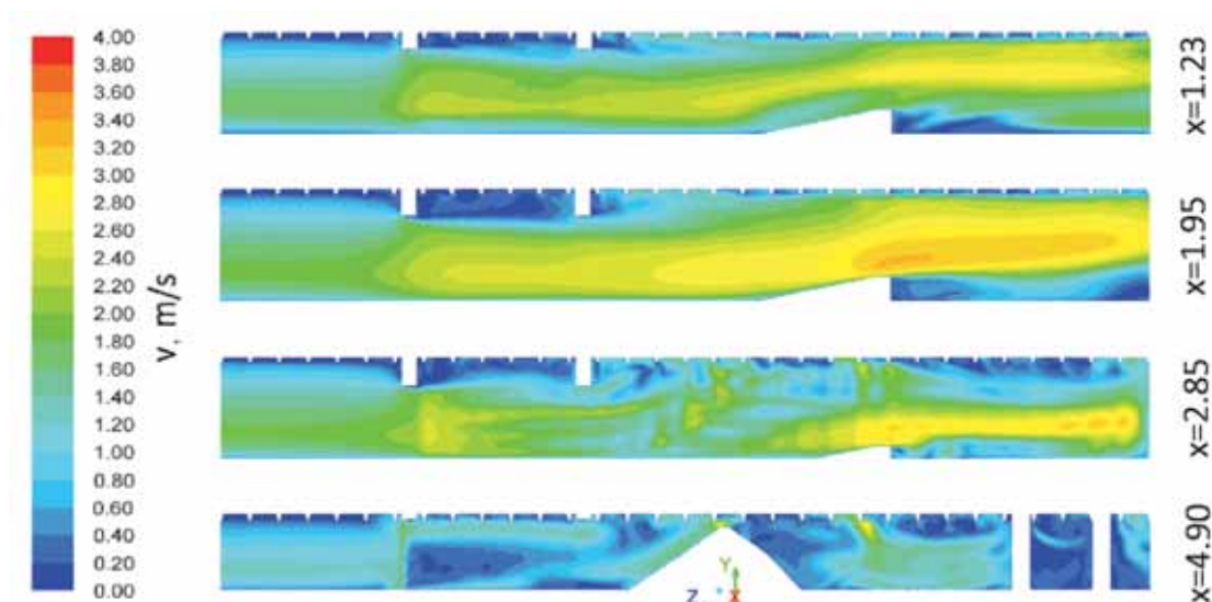
Rys. 19. Rozkłady prędkości w pionowych płaszczyznach równoległych do osi wyrobiska zawierających kolumny czujników monitorujących prędkość
