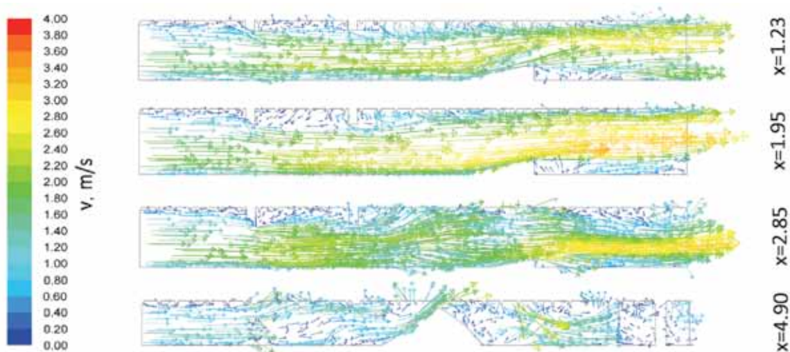
Rys. 20. Wektory prędkości w pionowych płaszczyznach równoległych do osi wyrobiska zawierających kolumny czujników monitorujących prędkość
