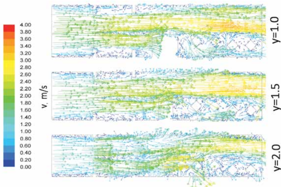
Rys. 18. Wektory prędkości na wysokościach 1, 1.5 i 2 m nad spągiem Fig. 18. Velocity vectors on 1, 1.5 and 2 m height under the floor
