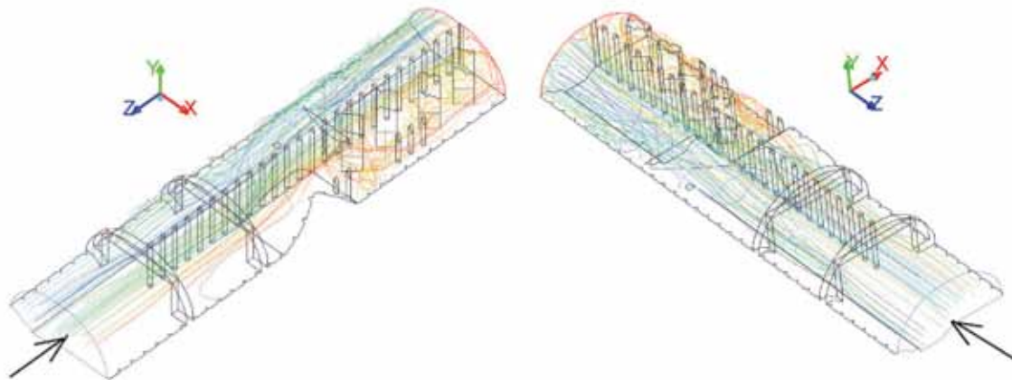
Rys. 14. Widok linii prądu dochodzących do przekroju wylotowego dla wariantu po ułożeniu przeszkody na spągu Fig. 14. View of velocity pathlines reaching the outlet section for the states after floor bulge
