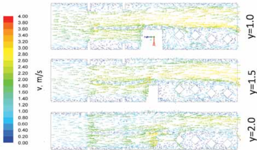
Rys. 10. Wektory prędkości na wysokościach 1, 1.5 i 2 m nad spągiem Fig. 10. Velocity vectors on 1, 1.5 and 2 m height under the floor
