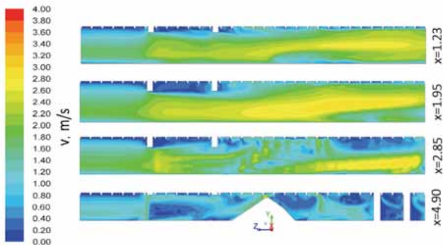
Rys. 11. Rozkłady prędkości w pionowych płaszczyznach równoległych do osi wyrobiska zawierających kolumny czujników monitorujących prędkość Fig. 11. Velocity distributions in vertical cross-sections parallel to the axis of mine drift containing velocity measurement points
