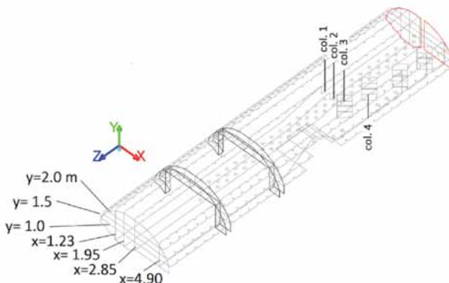
Rys. 7. Położenie powierzchni kontrolnych i linii pomiarowych w obszarze obliczeniowym
