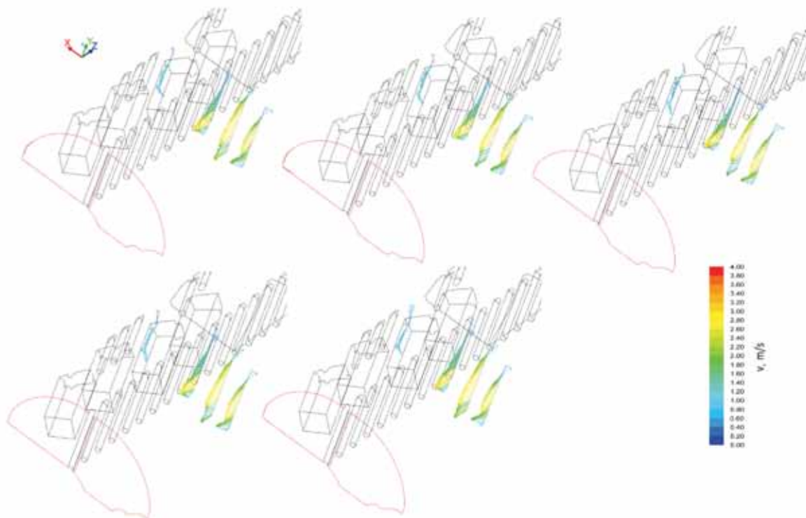
Rys. 13. Wektory prędkości na liniach zabudowy czujników anemometrycznych (Rys. 1) – obrazy co 2 sekundy symulacji
