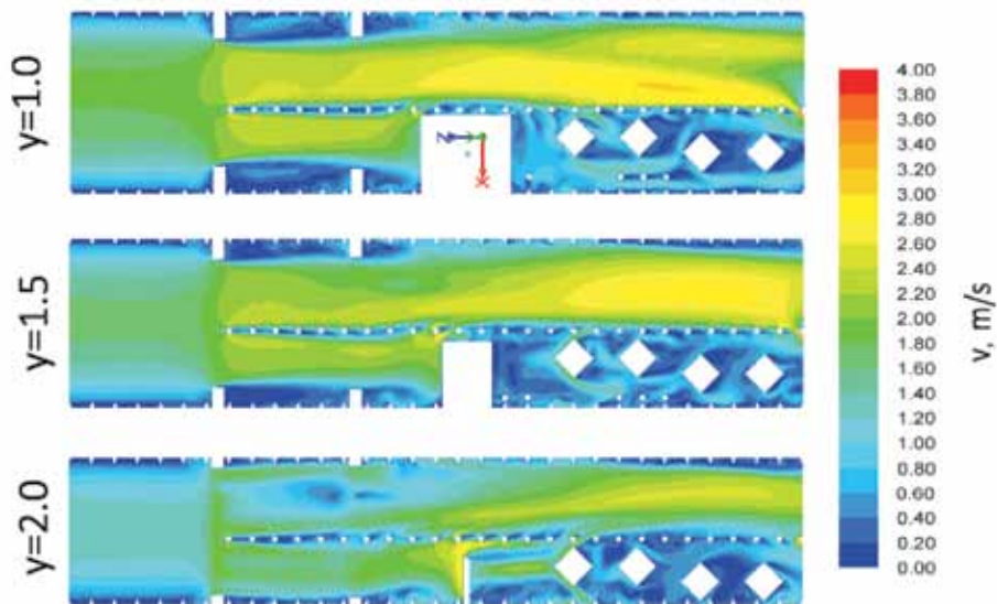
Rys. 9. Rozkłady prędkości na wysokościach 1, 1.5 i 2 m nad spągiem Fig. 9. Velocity distributions on 1, 1.5 and 2 m height under the floor
