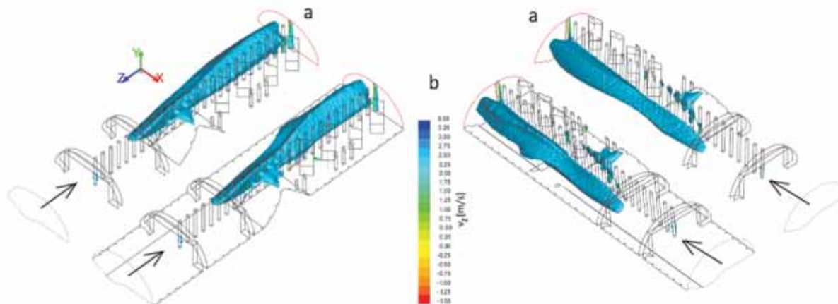
Rys. 16. Porównanie izopowierzchni prędkości 2.5 m/s, a - stan pierwotny, b - po ułożeniu przeszkody na spągu Fig. 16. Comparison of isosurface for 2.5 m/s velocity, a - state before, b - state after floor bulge
