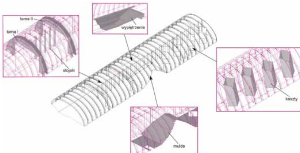
Rys. 2. Wybrane fragmenty geometrii obszaru Fig. 2. Selected fragments of the area geometry
