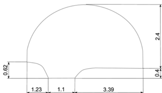
Rys. 4. Wymiary przekroju wlotowego i pomiarowego
