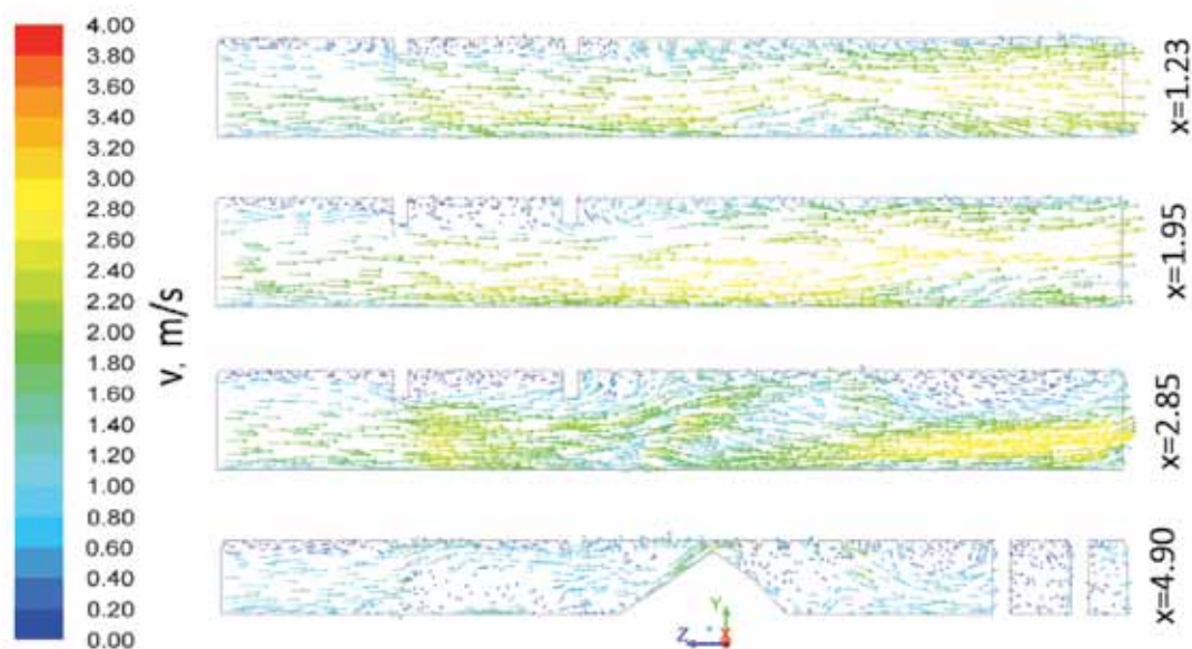
Rys. 12. Wektory prędkości w pionowych płaszczyznach równoległych do osi wyrobiska zawierających kolumny czujników monitorujących prędkość
