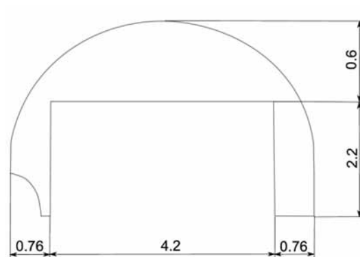
Rys. 5. Wymiary przekrojów w odrzwiach
