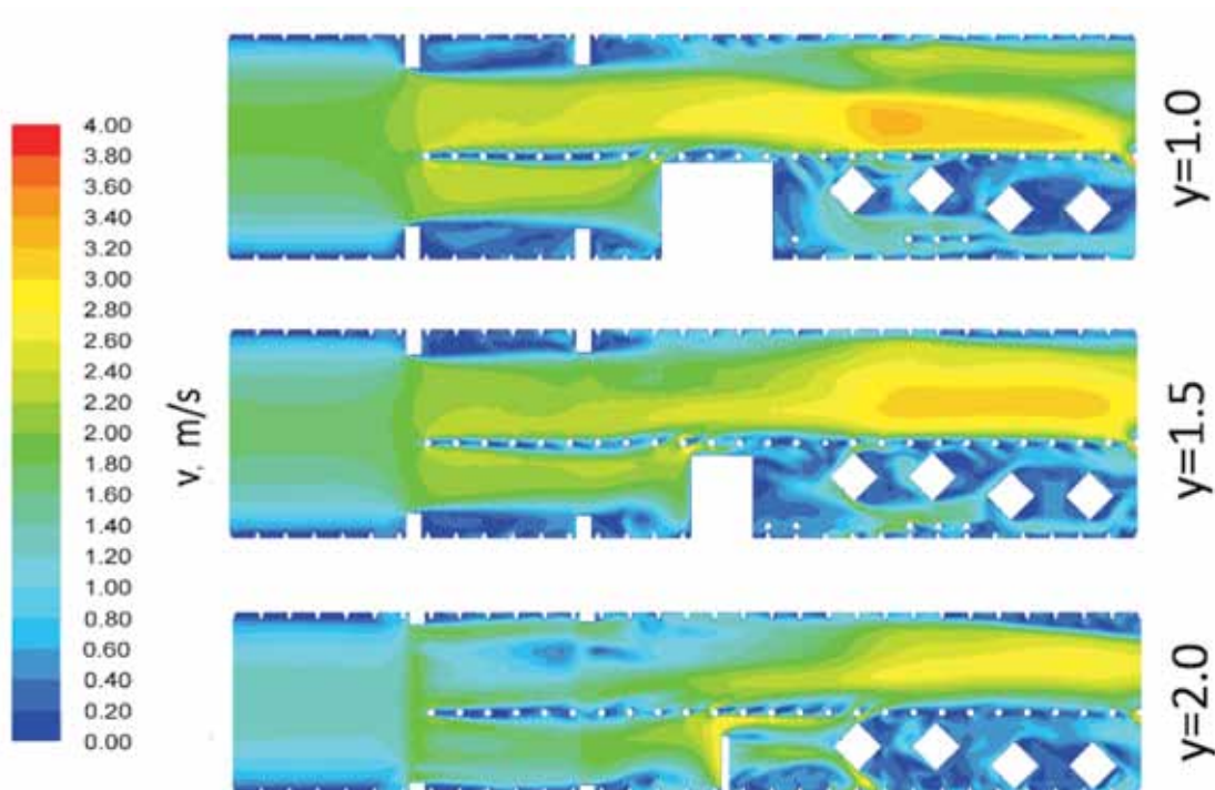
Rys. 17. Rozkłady prędkości na wysokościach 1, 1.5 i 2 m nad spągiem Fig. 17. Velocity distributions on 1, 1.5 and 2 m height under the floor
