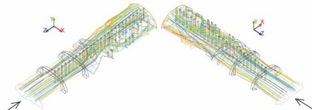
Rys. 8. Widok linii prądu dochodzących do przekroju wylotowego
