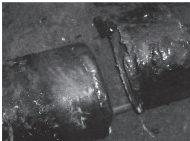
Rys. 10. Pęknięcie rurociągu stalowego w strefie rozciągania warstwy gruntu [4] Fig. 10. Crack of steel pipeline within the zone of soil layer loosening [4]
