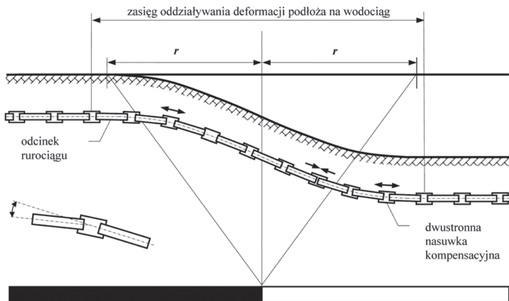
Rys. 3. Schemat oddziaływania górniczych deformacji podłoża wodociągu magistralnego z kompensatorami. Źródło: Opracowanie własne
