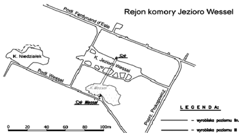
Rys. 1. Wyrobiska górnicze w rejonie Komory Jezioro Wessel Fig. 1. Mining excavations in the area of the Wessel Lake Chamber
