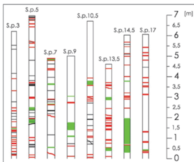
Rys. 1. Lokalizacja pęknięć i rozwarstwień skał stropowych w fazie utrzymania wyrobiska przyścianowego za frontem ściany 1/VI. szczelina; szczelina z rumoszem; pęknięcie.
