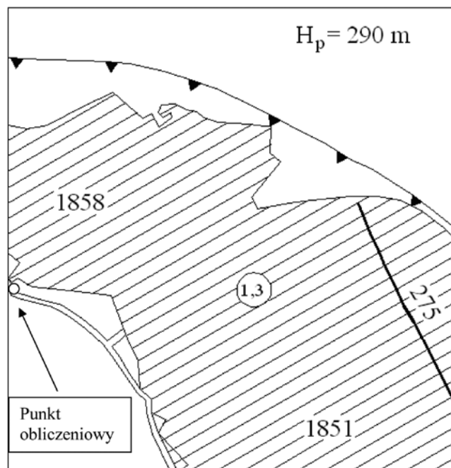
Rys. 1. Płytką eksploatacją w pokładzie 349/1 Fig. 1. Shallow exploitation in seam no. 349/1
