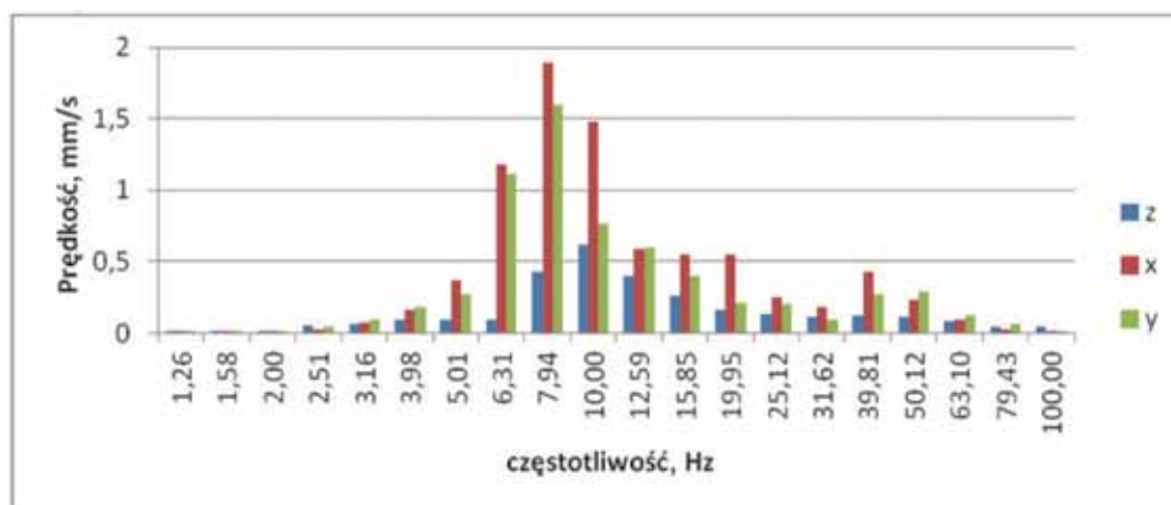
Rys. 3. Struktura częstotliwościowa drgań zarejestrowana na gruncie
