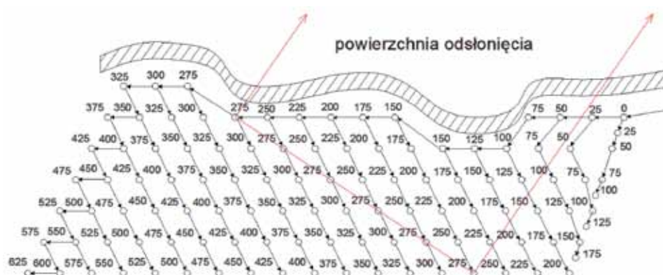
Rys. 1. Szescioszeregowy schemat odpalania przy użyciu zapalników nieelektrycznych [5]
