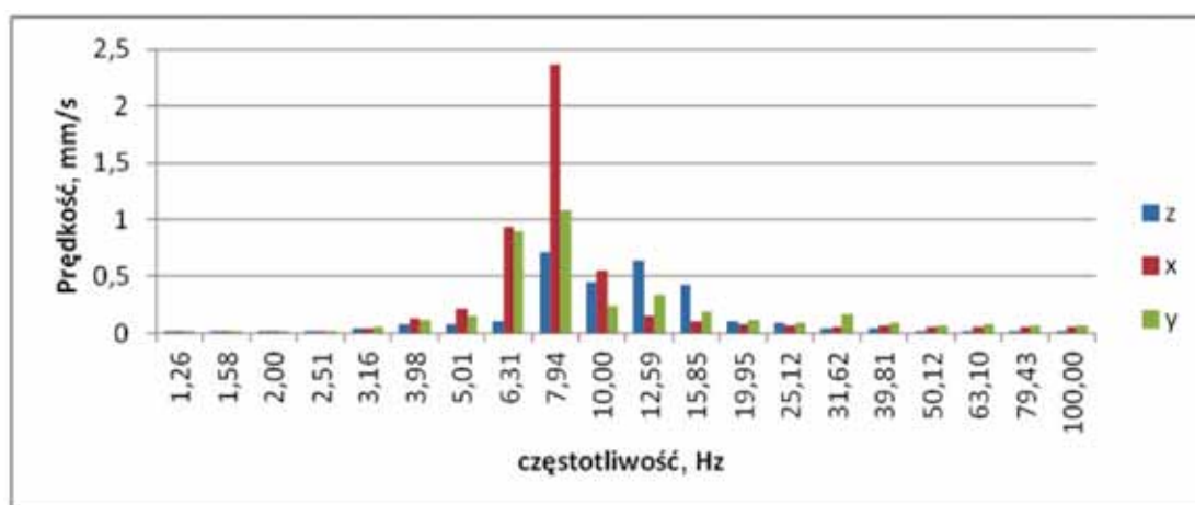
Rys. 4. Struktura częstotliwościowa drgań zarejestrowanych na fundamencie obiektu budowlanego
