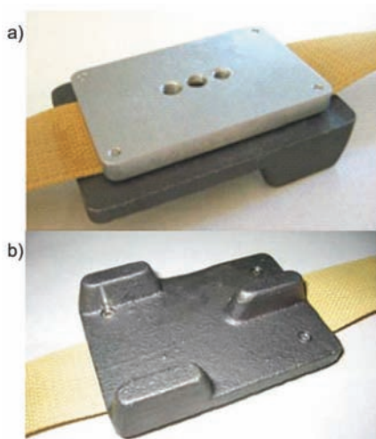
Rys. 4. LS-1: Górna płytką z gwintami pozwalającymi na montaż geofonów – a; dolna płytką podstawki – b [24]
