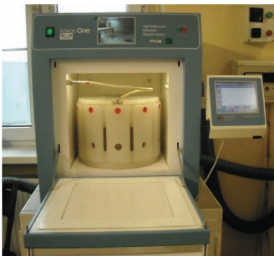
Rys. 1. Mineralizator wielostanowiskowy Ethos One Fig. 1. The mineralizator multiposition Ethos One
