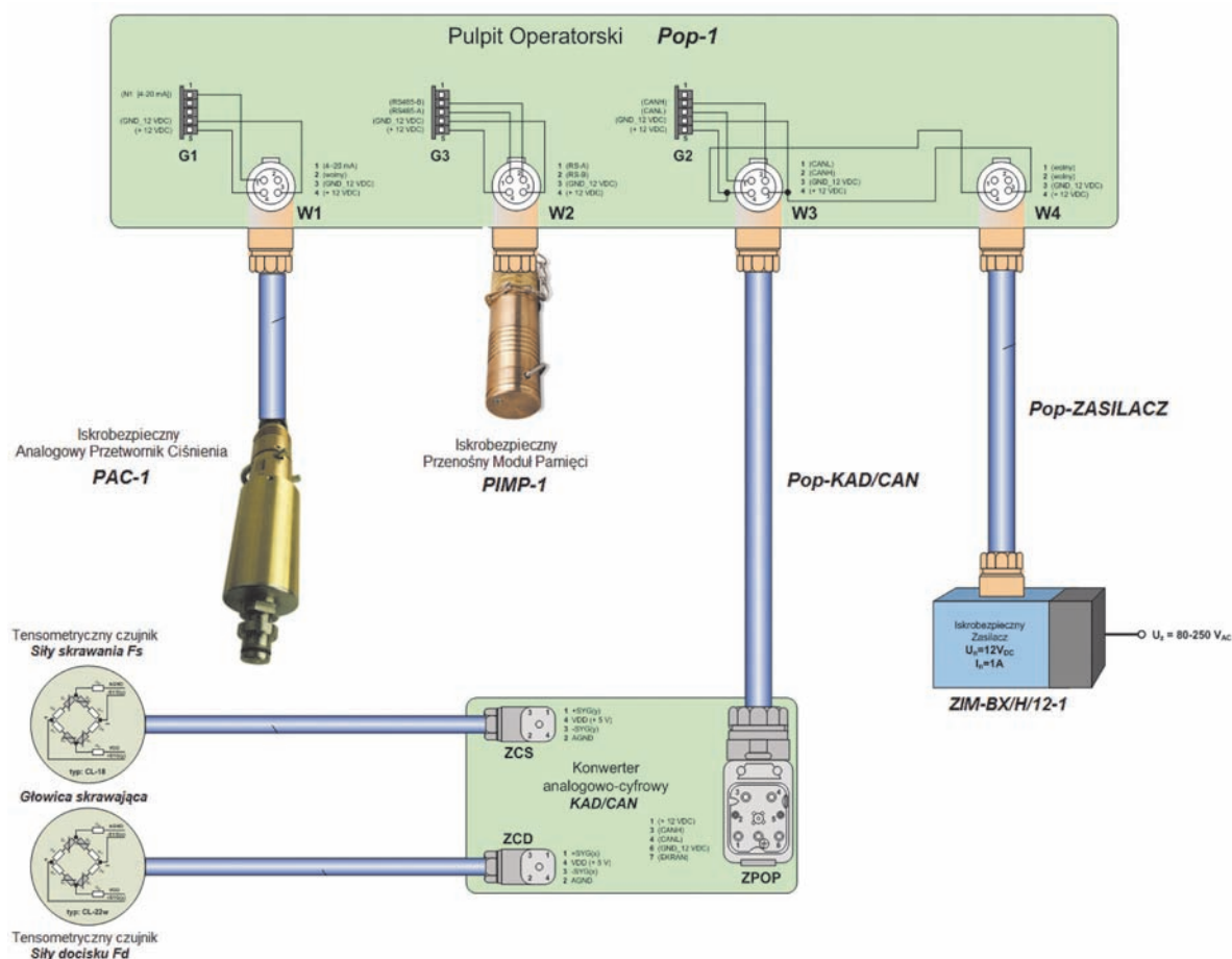
Rys. 3. Struktura układu PSSW
