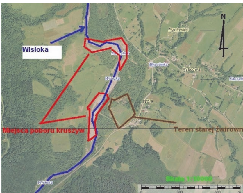
Rys. 4. Miejsca nielicencjonowanego poboru kruszyw z Wisłoki w Myscowej [opr. A. Kowalska] Fig. 4. Places of non-licensed exploitation of gravel in the Wisłoka river in Myscowa [el. A. Kowalska]
