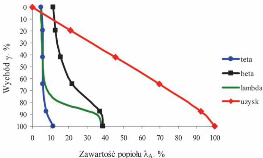
Rys. 2. Krzywa wzbogacania (zawartości popiołu) węgla z KWK Janina po wzbogacaniu w osadzarce ( \lambda – podstawowa krzywa wzbogalności rozkładu zawartości popiołu w badanym materiale, \nu – krzywa zawartości popiołu w koncentracie, \beta – krzywa zawartości popiołu w odpadzie, \varepsilon – uzysk części palnych i lotnych w koncentracie)
