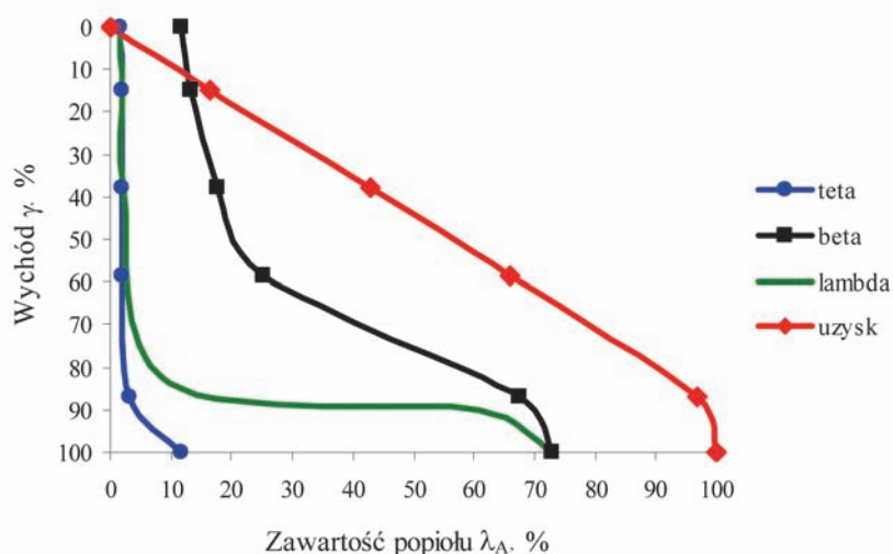
Rys. 3. Krzywa wzbogacania (zawartości popiołu) węgla z KWK Wieczorek po wzbogacaniu w osadzarce ( \lambda – podstawowa krzywa wzbogalności rozkładu zawartości popiołu w badanym materiale, \nu – krzywa zawartości popiołu w koncentracie, \beta – krzywa zawartości popiołu w odpadzie, \varepsilon – uzysk części palnych i lotnych w koncentracie).
